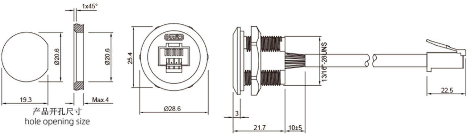
尺寸图
