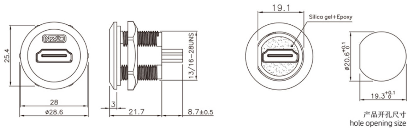
尺寸图
