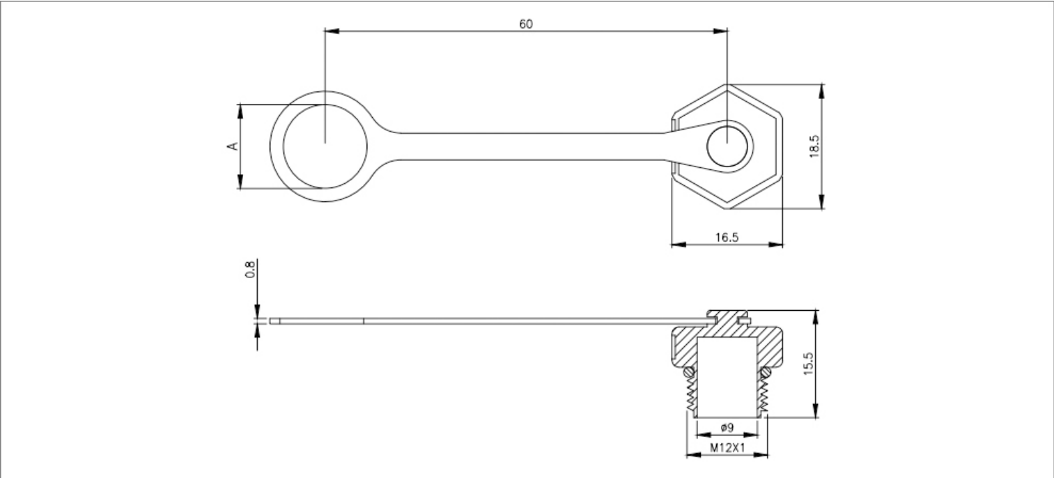
尺寸图
